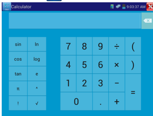
Рис. 3.3.20-1 Калькулятор
