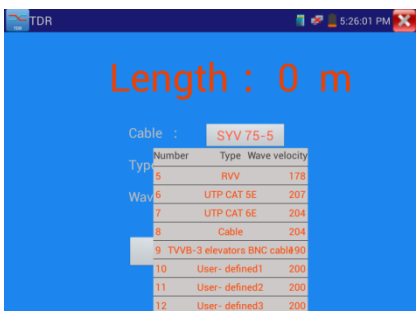
Рис. 3.3.19-5 Выбор кабеля
